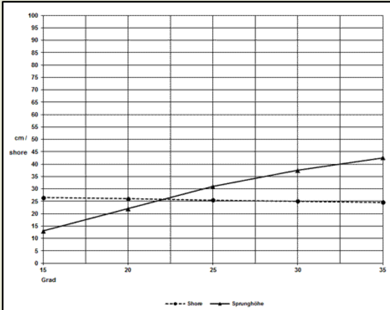
Diagramm 1 (414), zeigt die Abhängigkeit von Sprunghöhe und Härte zur Temperatur
