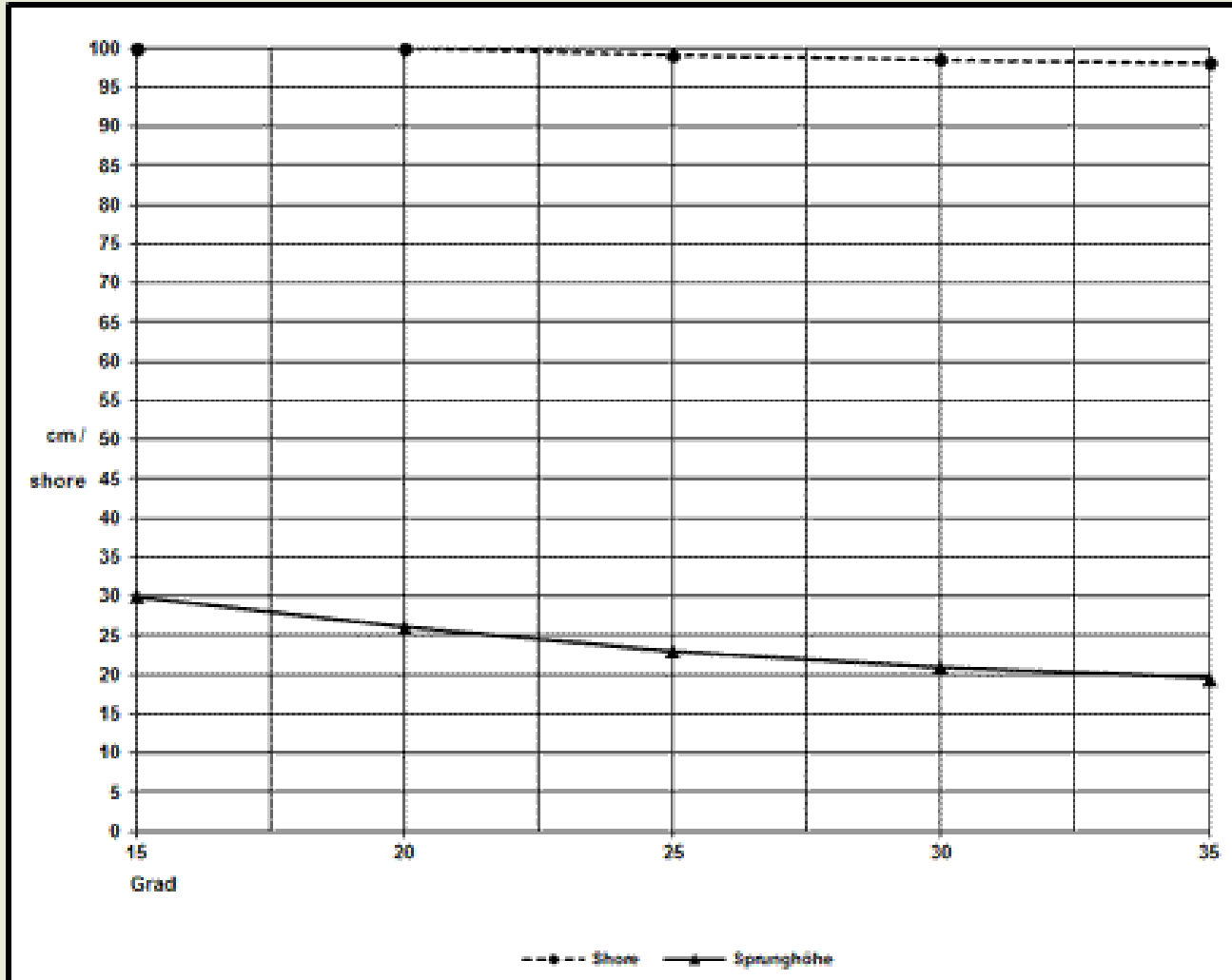
Diagramm 2 (593), zeigt die Abhängigkeit von Sprunghöhe und Härte zur Temperatur
